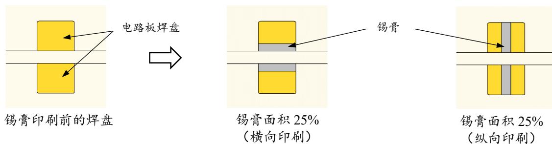
图 11. 试验品的锡膏印刷方法例
