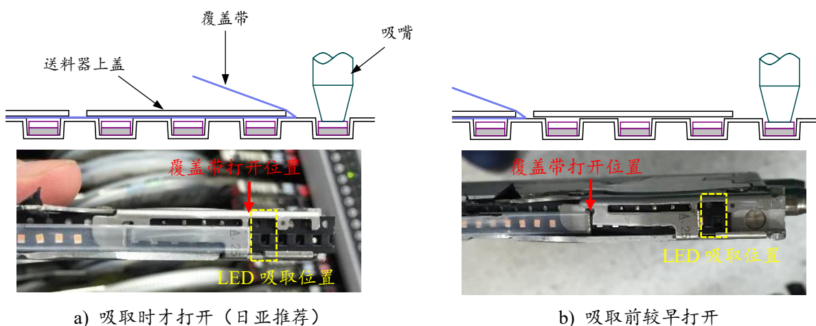
图 17. 覆盖带打开位置
