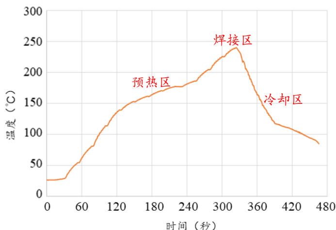
图 24. 回流焊温度曲线例
