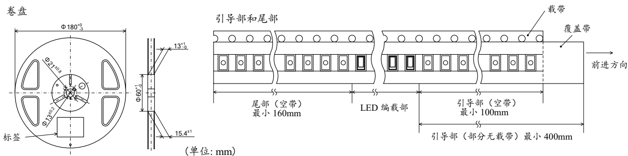
图 1. 卷盘和编带（例：NC2x170x 规格书摘抄）
