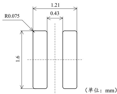
图 7. 电路板焊盘和网版开口推荐（例：NCSx170x 规格书摘抄）
