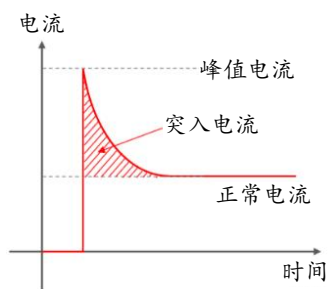
图 28. 突入电流曲线例
