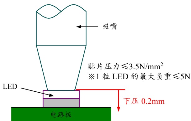
图 22. 推荐贴放高度
