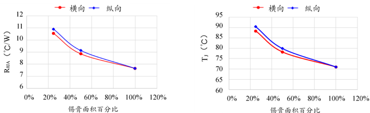
图 12. 不同锡膏面积下的 R_{0JA} 和 T_J (实测值)
