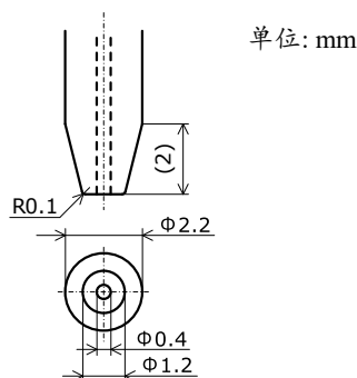
图 13. 日亚推荐吸嘴
