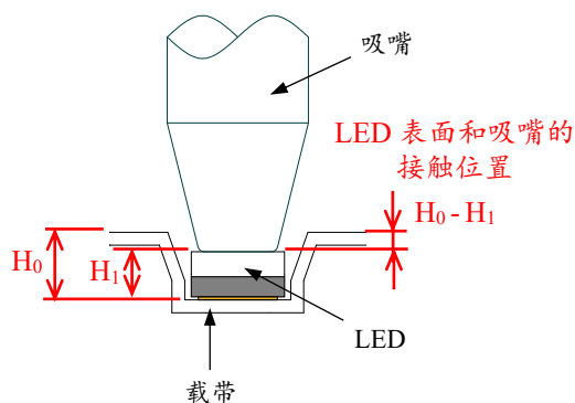
图 15. 推荐吸取高度
