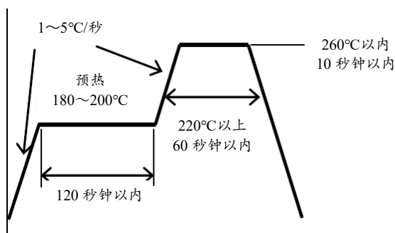
图 23. 回流焊条件（使用无铅锡膏时）
