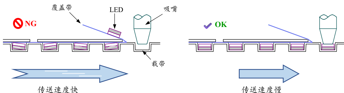
图 20. 送料器的传送速度
