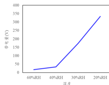
图 19. 湿度 vs. 带电量
