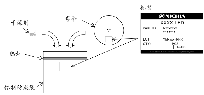
图 2. 铝制防潮袋
