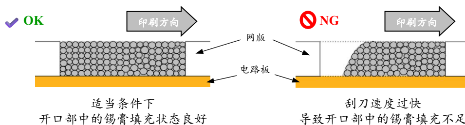
图 8. 刮刀速度和网版开口部的锡膏填充状态
