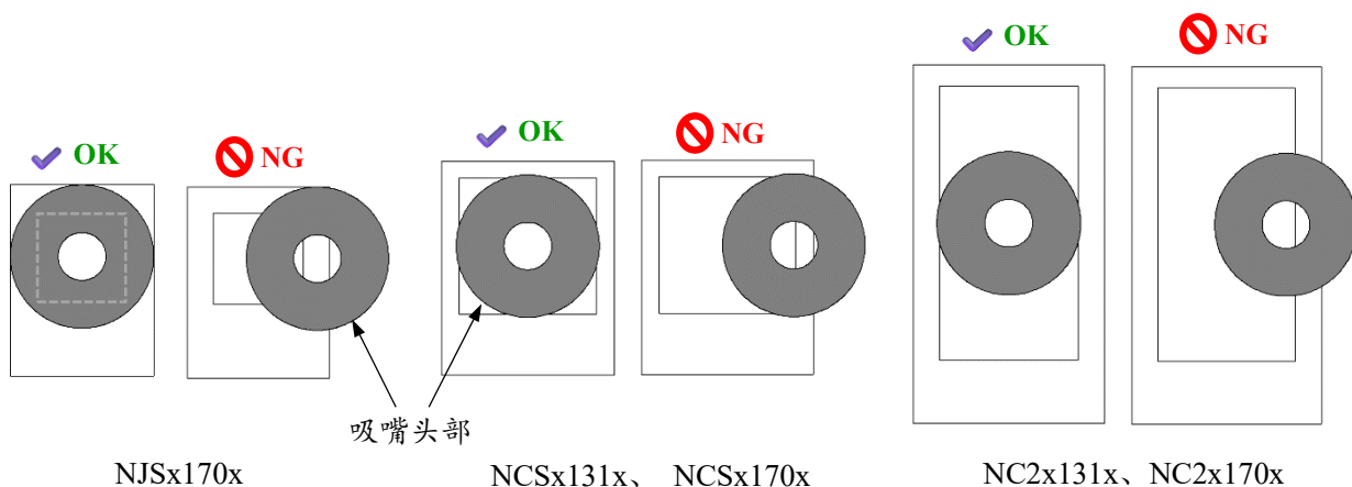
图 14. 吸嘴吸取位置
