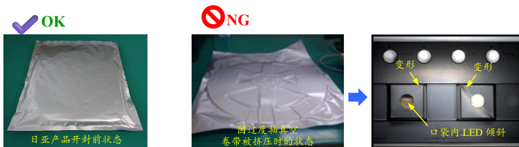
图 6. 过度抽真空导致的载带变形
