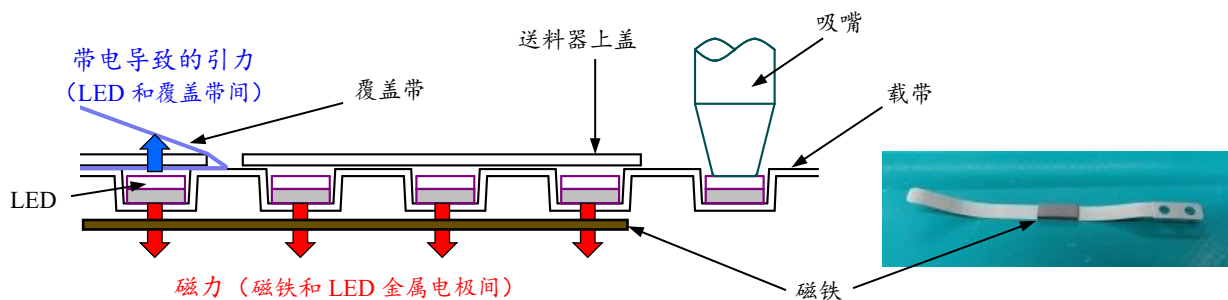
图 21. 送料器下方的磁铁
