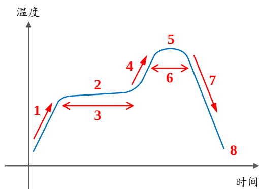
图 25. 回流焊温度曲线调整位置
