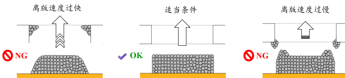
图 9. 网版的离版速度和锡膏形状
