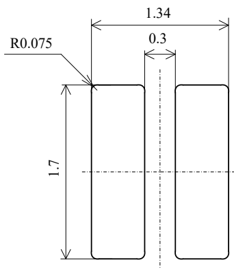
图 7. 电路板焊盘和网版开口推荐（例：NCSx170x 规格书摘抄）
