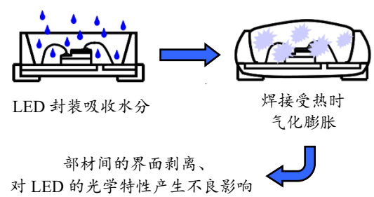
图 3. LED 的受潮和气化膨胀示意图
